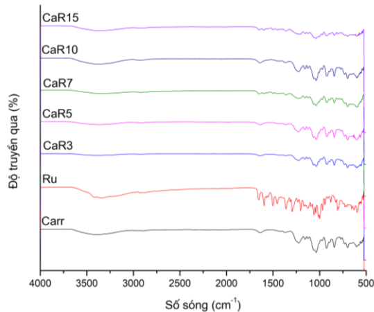
Hình 2. Phổ FTIR của Carr, Ru và CaR
